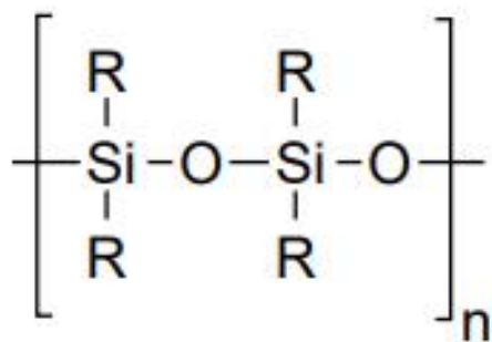
Vzorec silikonu
