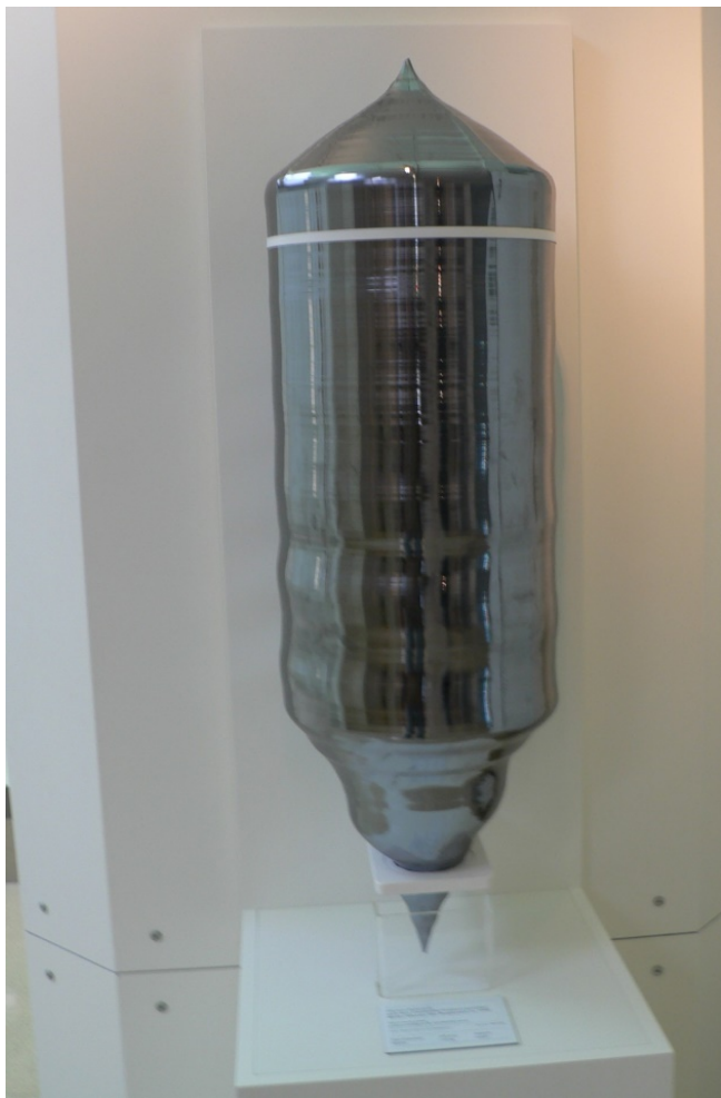
Krystal křemíku
