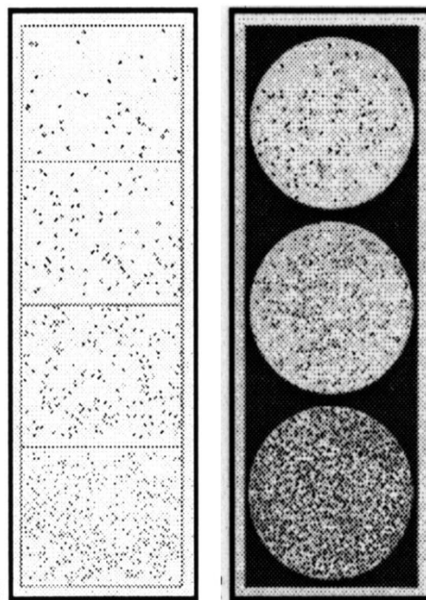
Obr. 2.: Výškové rozložení brownovských částic ve vodní suspenzi (převzato z [23])
