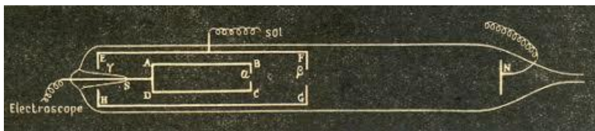
Obr. 1.: Perrinova katodová trubice (převzato z [1])
