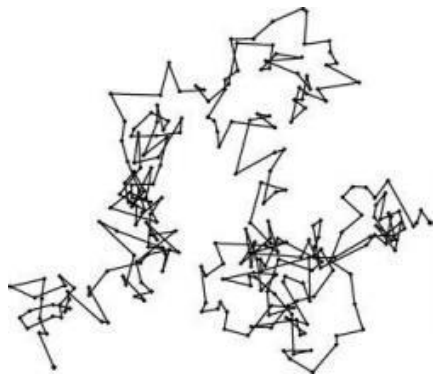
Obr. 3.: Periodický záznam poloh vybrané brownovské částice
